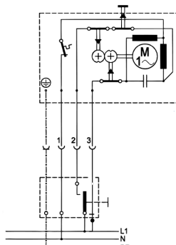
Drives/ Antriebe: D239 | D249 | D259 | D339 D349 | D359 | D539 | D839
