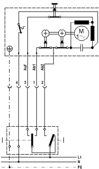
Drives/ Antriebe: D248 | D258 | D348 | D358 D838
